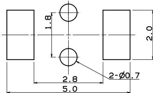
P.C.B DIMENSION
